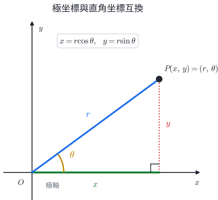
圖 1-4：極坐標與直角坐標互換。點 P 既可記為直角坐標 (x, y) ，也可記為極坐標 (r, \theta) ，兩者由 x = r \cos \theta 、 y = r \sin \theta 相連。
